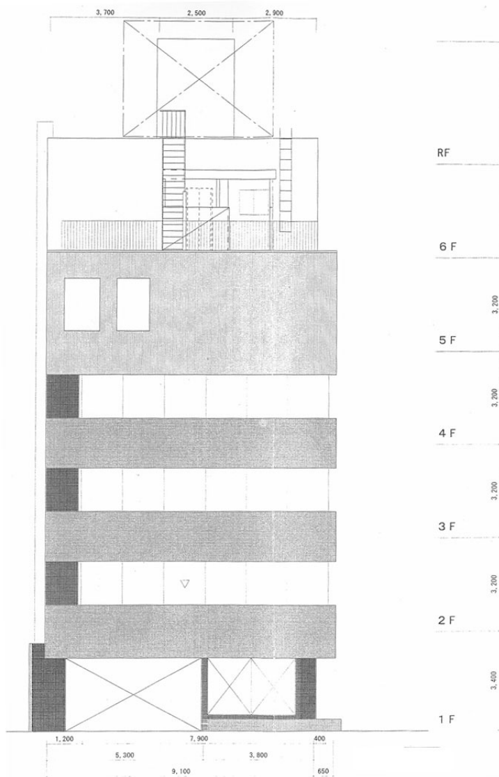
東立面図
