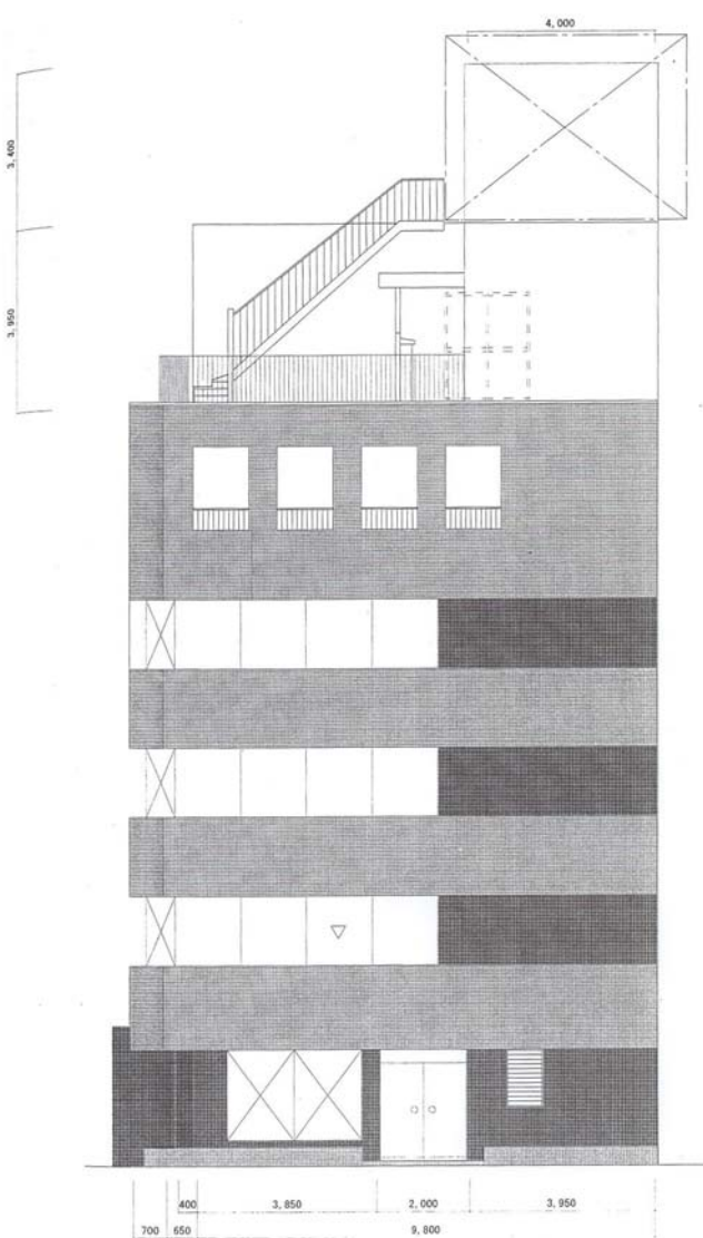
北立面図
